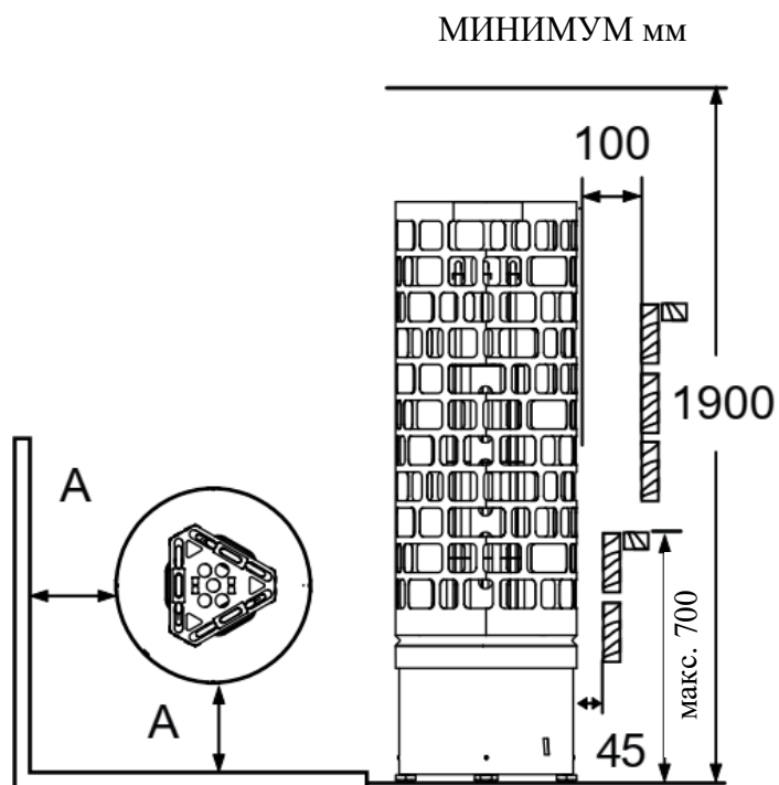
Рис. 2 Минимальные безопасные расстояния (мм)
