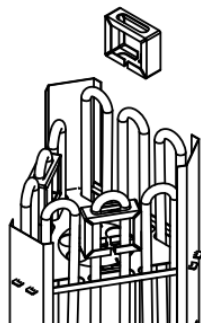
Рис. 3 | Разделитель нагревательных элементов
